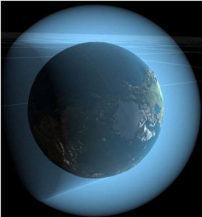
Рис.14 Атмосфера Земли
