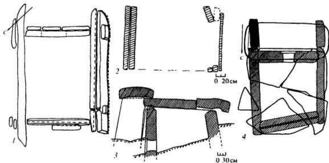
Рис. 3. Археологические памятники из района г. Туапсе. 1, 2 – пос. Новомихайловский. Гробница на р. Псыбэ (план без погребений и продольный разрез. По М.К. Тешеву); 3, 4 – пос. Анастасевка уроч. Адигналово. Портальный дольмен № 8 (продольный разрез и план. Обмеры В.И. Марковина)
