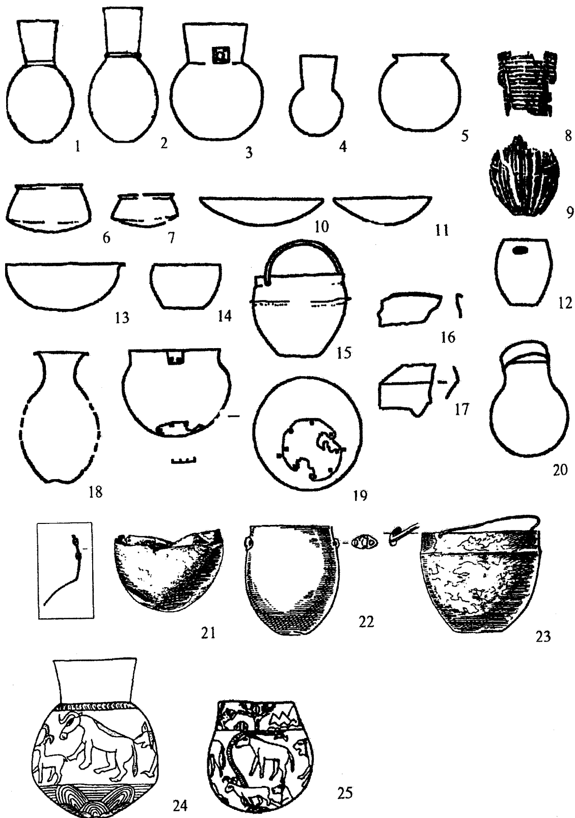
Рис. 1. Металлическая посуда галюгаевско-серегинского варианта майкопско-новосвободненской общности. 1-18,21,24-25 – Майкопский курган; 19 – п.70 в к.1 у с.Заманкул; 20 – Старомышастовский клад (21-23 – рисунки сосудов Майкопского кургана по Ю.Ю.Пиотровскому). Серебро – 1,3-6,8-10,12-14,20,24,25. Золото – 2,7. Бронза – 11,15-17,21-23
