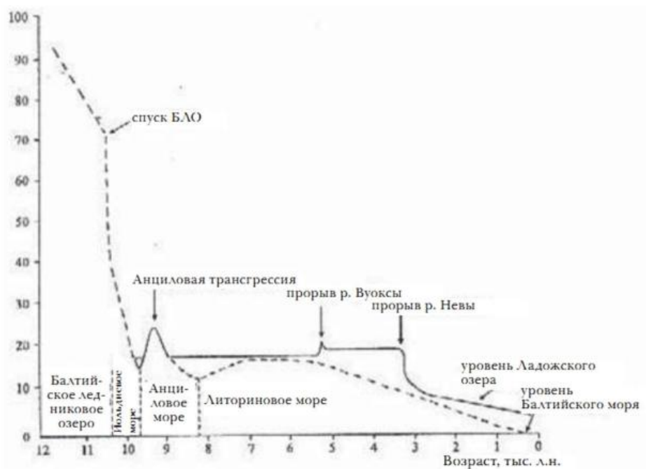
Рис. 7. Реконструкция изменений уровней Ладожского озера и Балтийского моря в поздне- и послеледниковые
