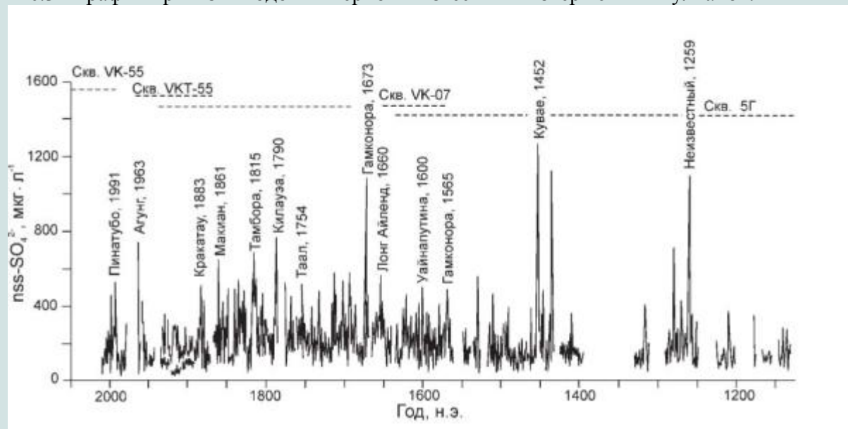
Рис.32 График привязки годовых кернов к известным извержениям вулканов.
