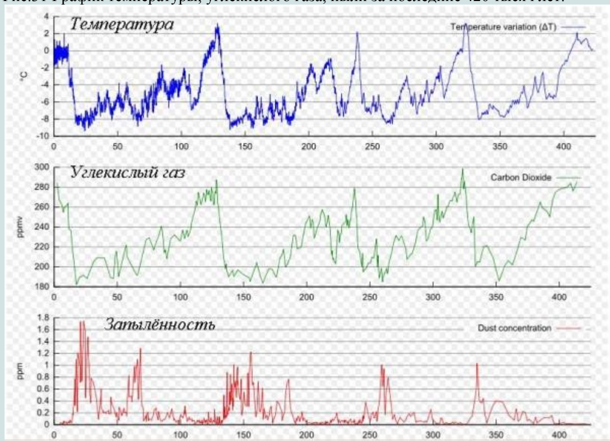
Рис.31 График температуры, углекислого газа, пыли за последние 420 тысяч лет.
