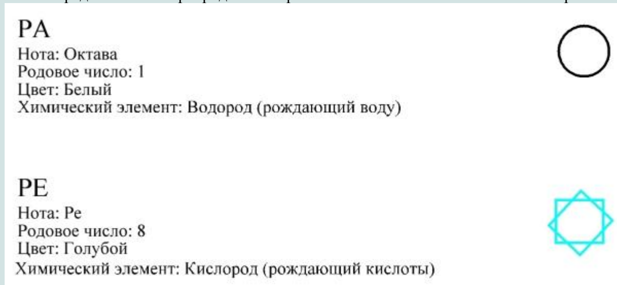
Рис.11 Представление первородного энергетического потока РА и октавной энергии РЕ.
