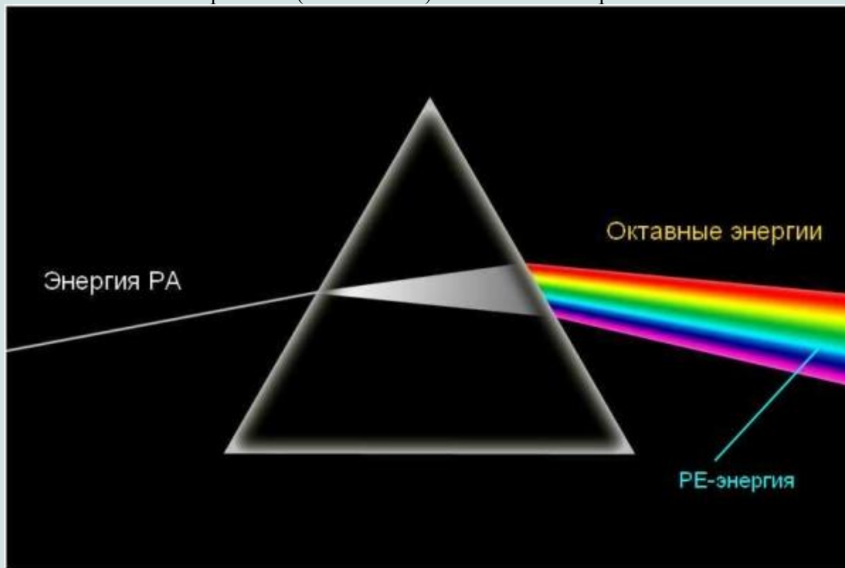
Рис.9 Разложение энергии РА (белого света) на Октавные энергии.
