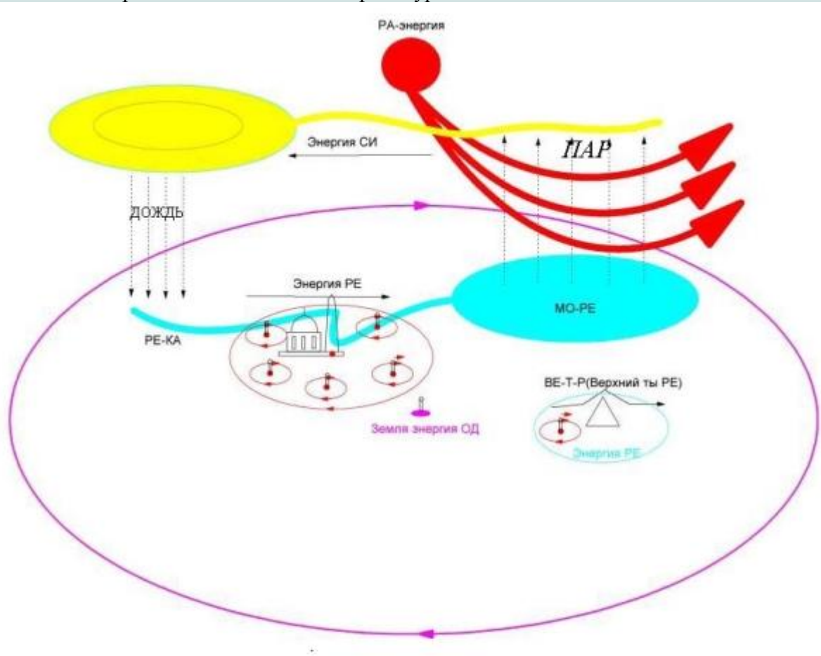
Рис.13 РЕ-энергия естества на планетарном уровне.
